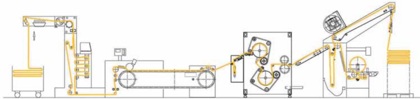
Comptex RC: compacting machine for open width fabrics. Comptex RC: máquina compactadora por tejidos en abierto. Comptex RC: máquina compactadora por tecidos em aberto.
